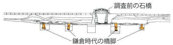
称名寺苑池の断面図（部分）
